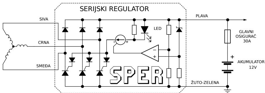
Slika 2 - Spoj regulatora (5/7 žica):
