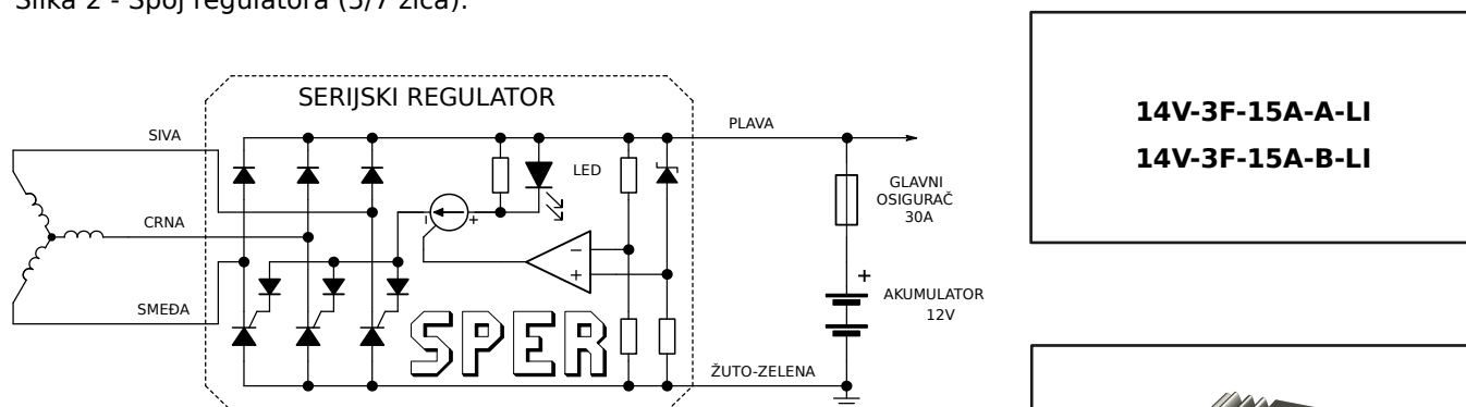
Slika 2 - Spoj regulatora (5/7 žica):
